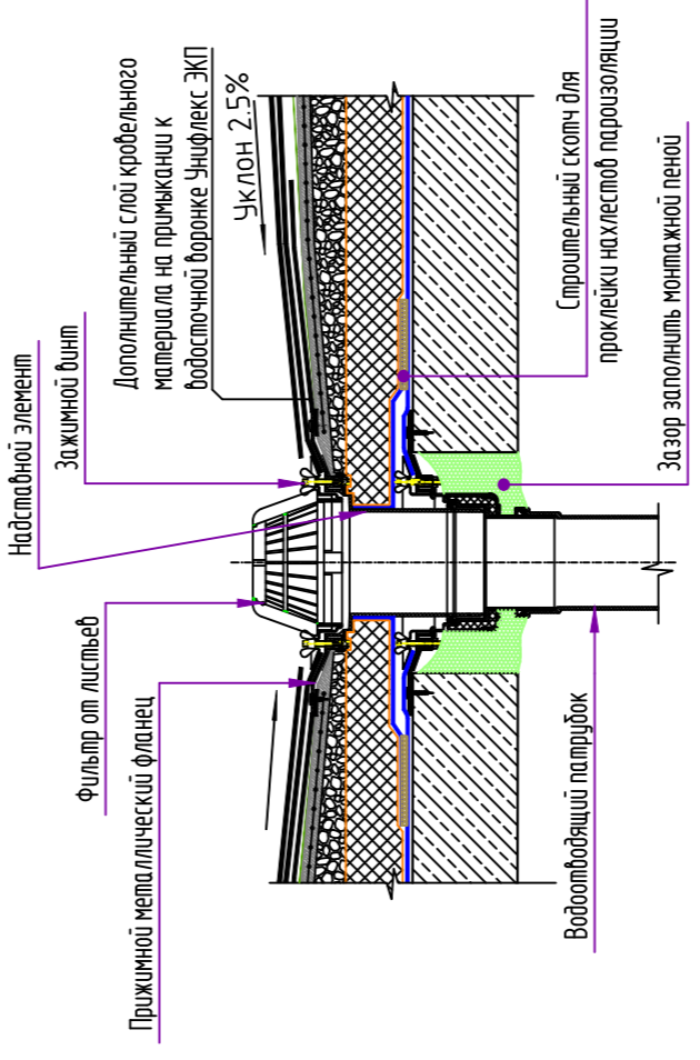
Узел устройства водосточной воронки
